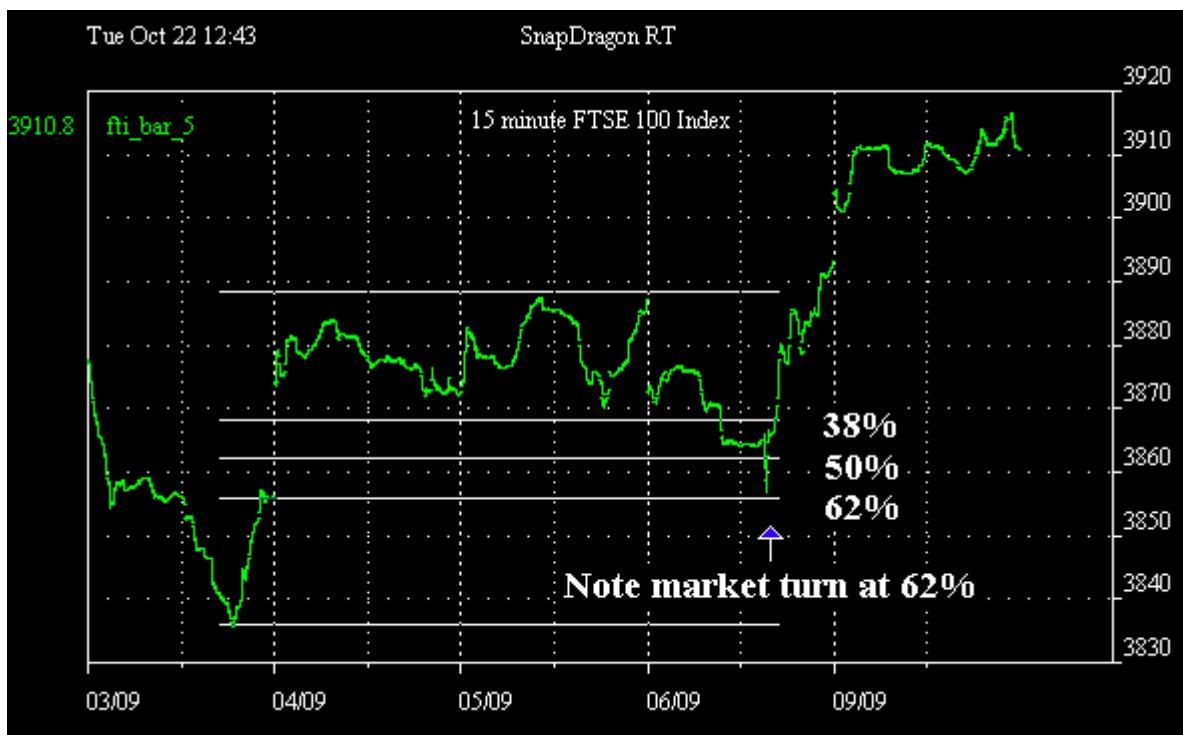
6 pav. Fibonacci lygiai
